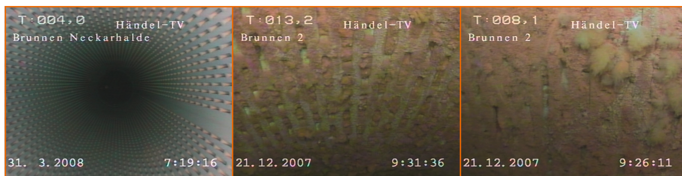
obere Reihe: links: intakter Brunnenfilter ohne Ablagerungen, mitte: stark zugesetzter Brunnenfilter, rechts: Detailausschnitt mit Algen- und Bakterienwachstum im Brunnen
