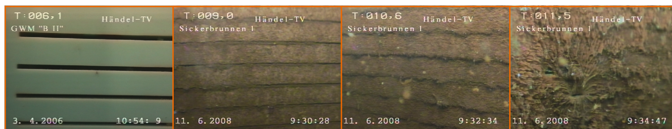
untere Reihe: links: Detailausschnitt eines sauberen Brunnenfilters, mitte: zunehmende Verkeimung und Verockerung eines Brunnenfilters, rechts: Detailblick auf massiven Biofilm auf Brunnenfilter
